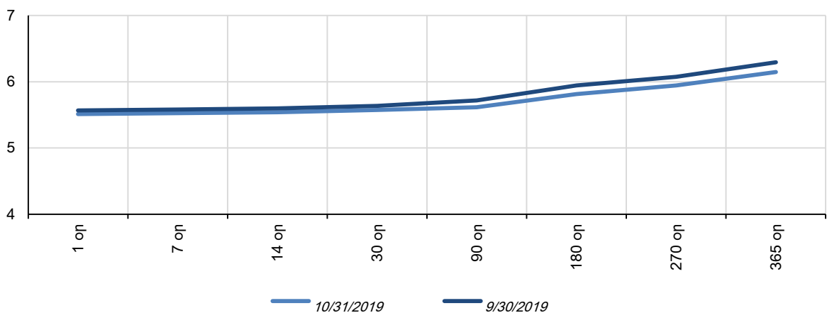
Ջեդճատոկոսային պարտատոմսերի եկամտաբերության կոր
